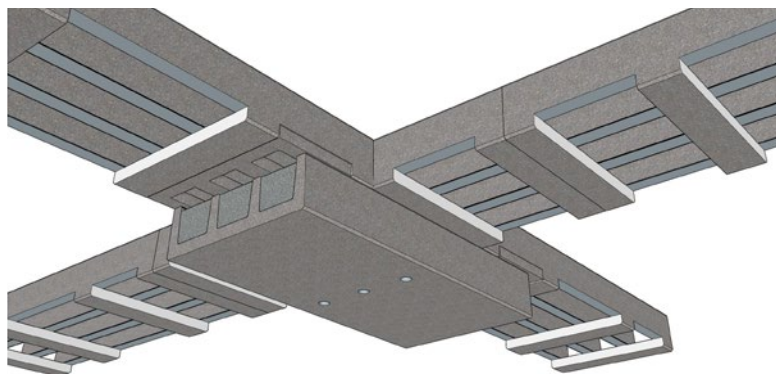
KABELKORSNING med undergående kanal med avfasade kabelövergångskanter.
